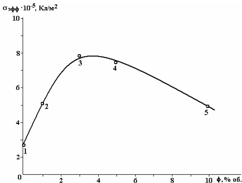
Рис. 1. Зависимость поверхностной плотности заряда короноэлектретов из полимерной композиции ПЭНП+х об.% TlInSe 2 (где х: 1–0; 2–1; 3–3; 4–5; 5–10) от объемного содержания наполнителя
