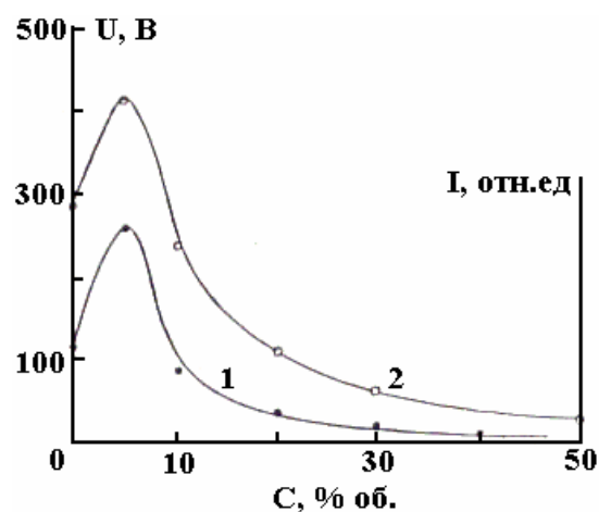
Рис. 3. Зависимости интенсивности пика стеклования (кривая 1) и стабилизированной электретной разности потенциала (кривая 2) коронозэлектретов композита ПЭВП + фиброин. Поглощенная доза – 1 \cdot 10^4 Гр.; режим поляризации U_n = 7 кВ, t_n = 300 с
