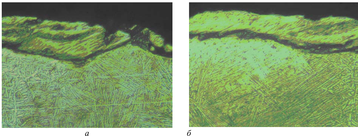
Рис. 5. Микроструктура образца титанового сплава BT20, подвергнутого электроискровому легированию без предварительной пассивации поверхности графитом (а) и при пассивации ее в режиме энергии разряда 0,3 Дж (б). \times 500
