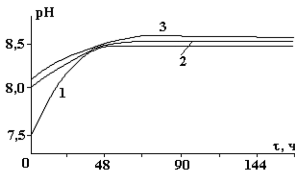
Рис. 2. Влияние продолжительности испытаний на pH среды при концентрации ингибитора, г/л: 1 – 0; 2 – 0,25; 3 – 0,5
