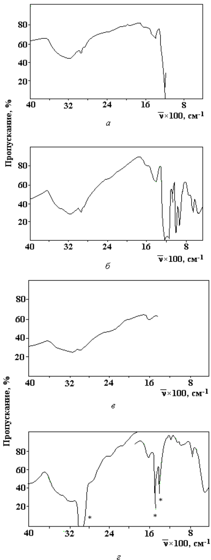
Рис. 9. ИК-спектры поглощения во фторированном (а – в) и вазелиновом масле (г) продуктов коррозии стали Ст.3 в воде + 0,5 г/л Thsc (а,б) и осадка со дна стакана (в,г) при времени выдержки, час: а – 48; б, в, г – 168
