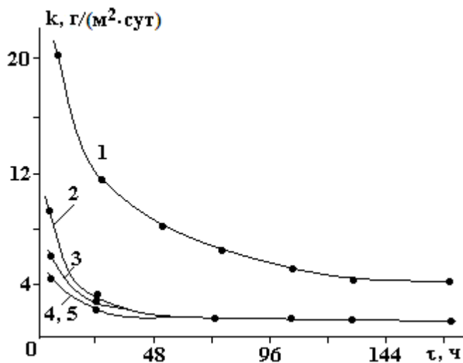
Рис. 1. Влияние продолжительности испытаний на скорость коррозии при концентрации ингибитора, г/л: 1 – 0; 2 – 0,25; 3 – 0,4; 4 – 0,45; 5 – 0,5
