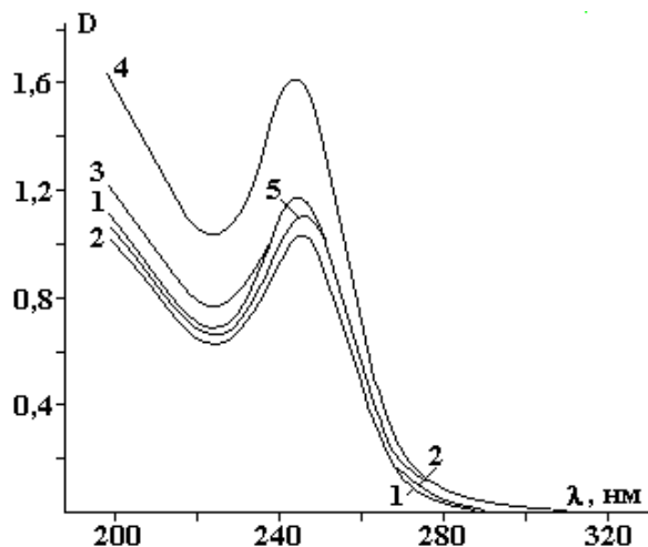
Рис. 5. УФ-спектры поглощения воды с добавкой 0,5 г/л Thsc при времени коррозии стали Ст.3, ч: 1-0; 2-24; 3-48; 4-72; 5-288
