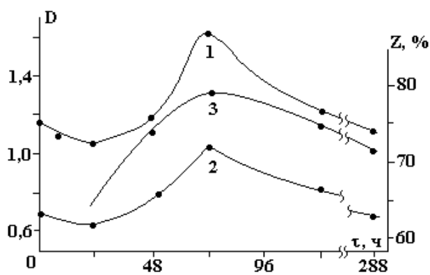
Рис. 6. Влияние времени испытаний на интенсивность поглощения коррозионной среды (вода +0,5 г/л Thsc) в максимуме кривой поглощения (1) и ее минимуме (2) (см. рисунок 5) и степени защиты (3)
